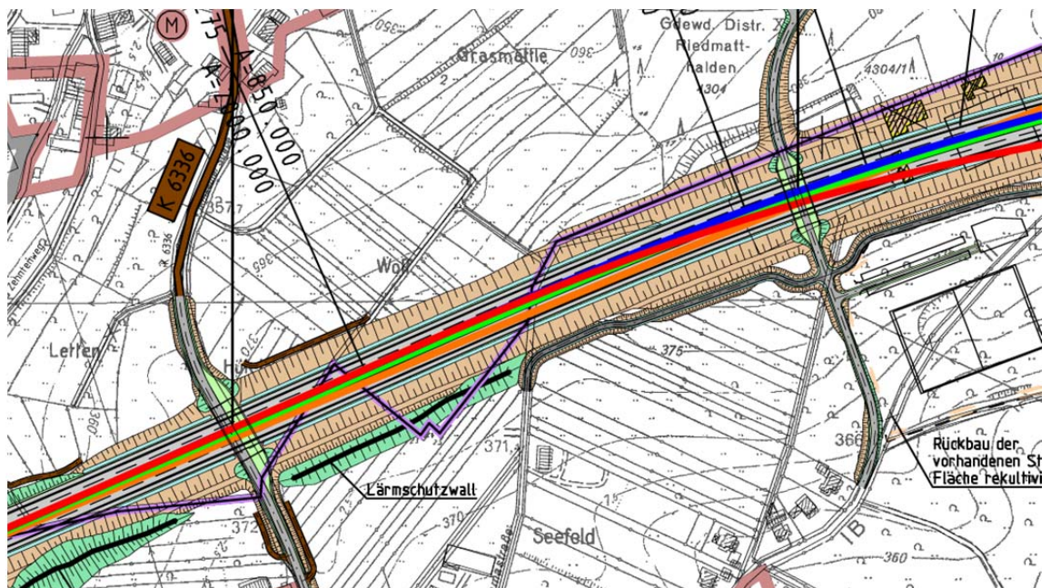
Abbildung 7: Ausschnitt aus Lageplan Variante 2 Unterlage 1.2 Blatt 2.1
