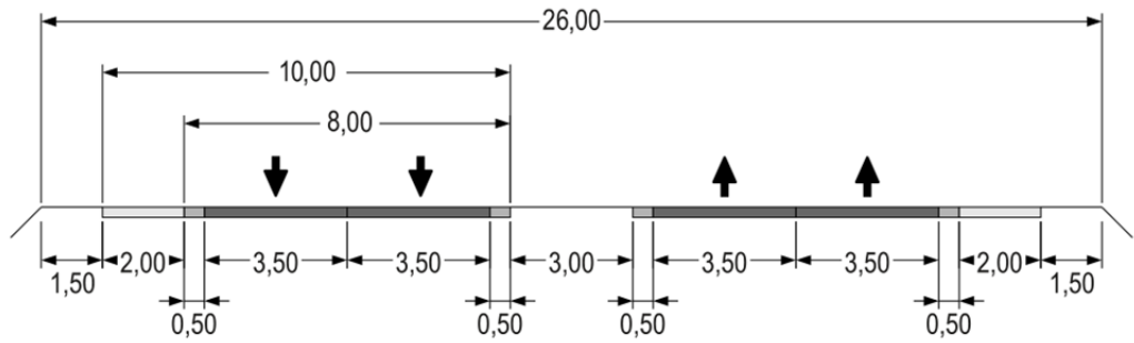
Abbildung 12: RQ 26 gemäß RAS-Q 1996
