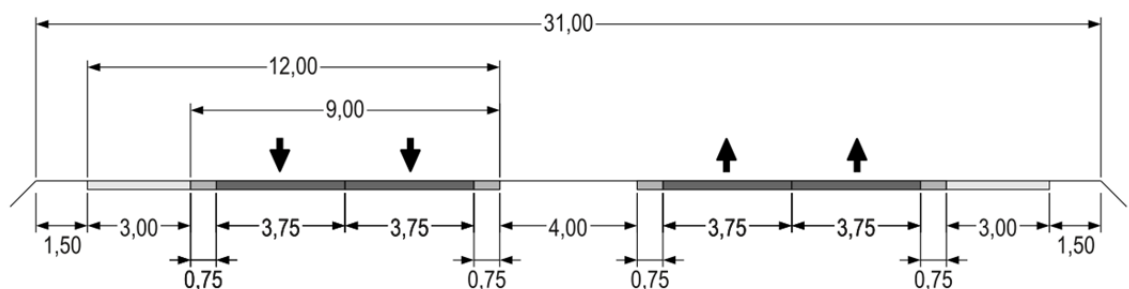
Abbildung 11: RQ 31 gemäß RAA 2008
