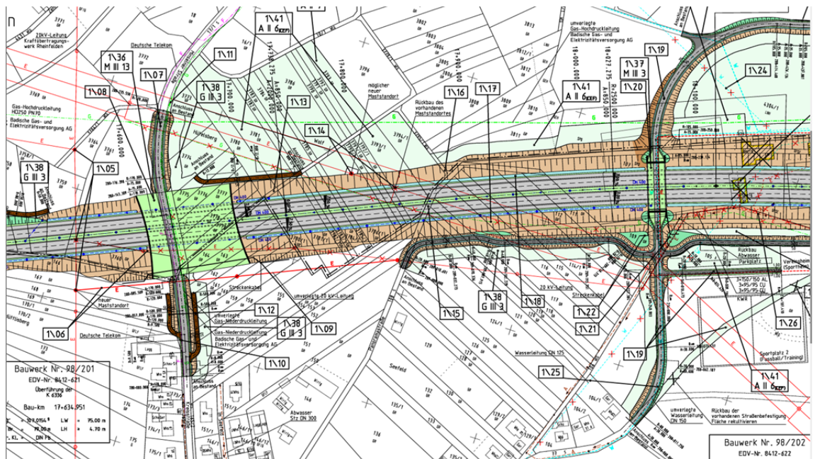
Abbildung 1: Ausschnitt als Lageplan Unterlage 5 Blatt 1
