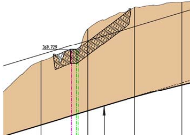
Abbildung 3: Ausschnitt aus Höhenplan Unterlage 6 Blatt 1
