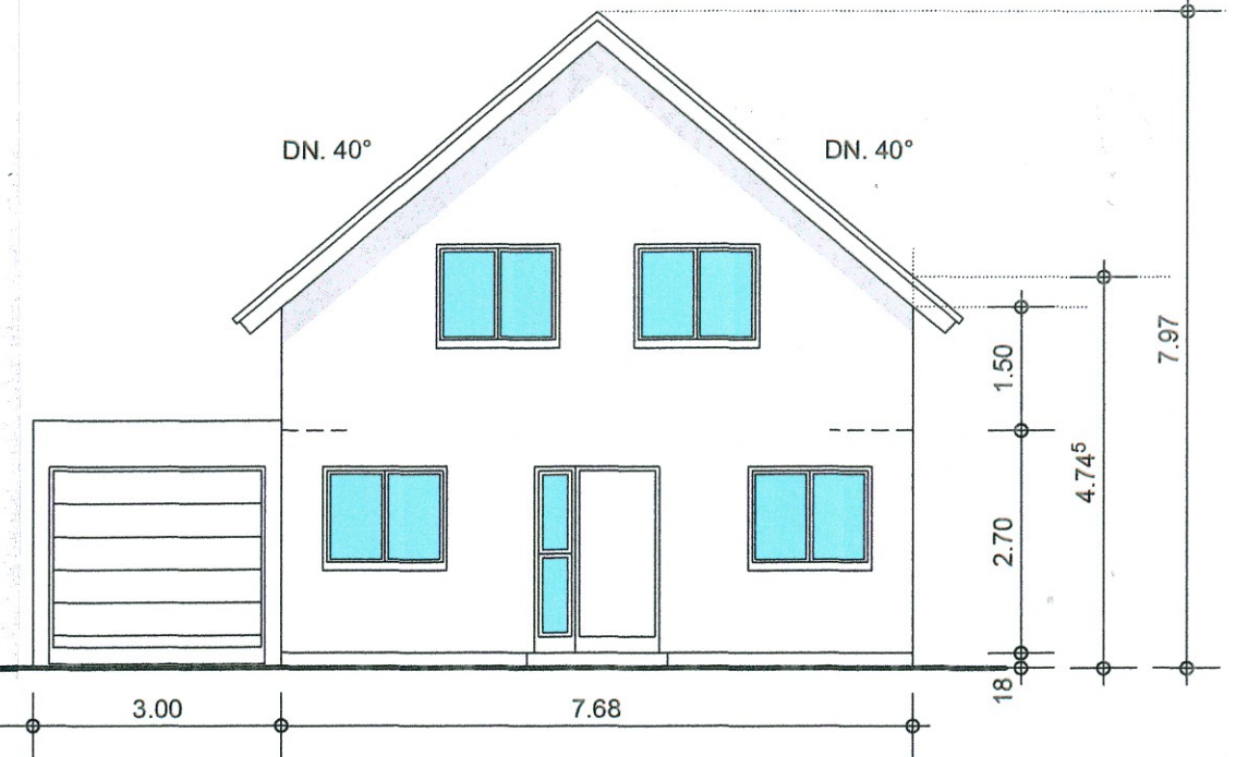
WESTEN M.1:100
