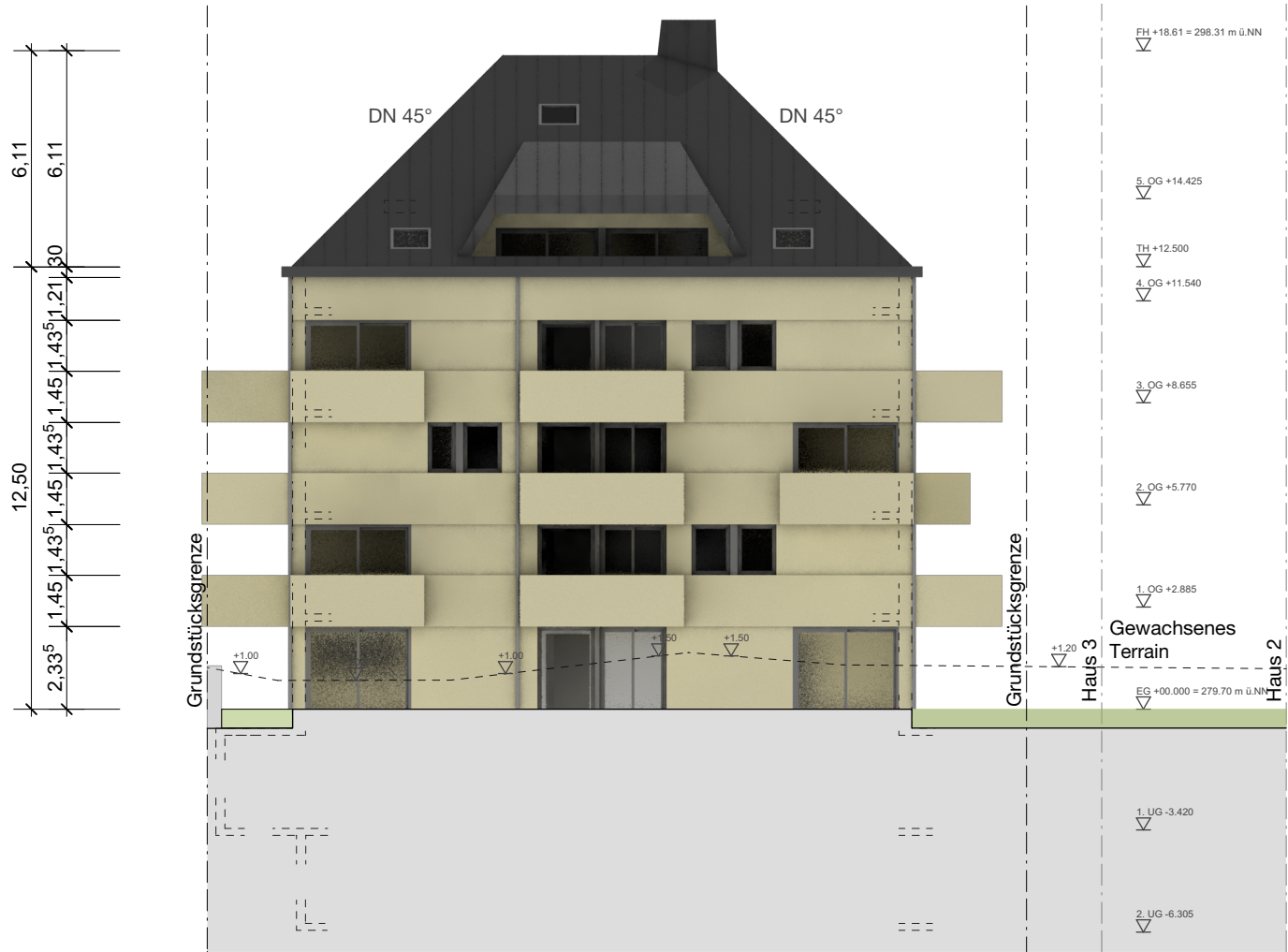
HAUS 1 ANSICHT OST
