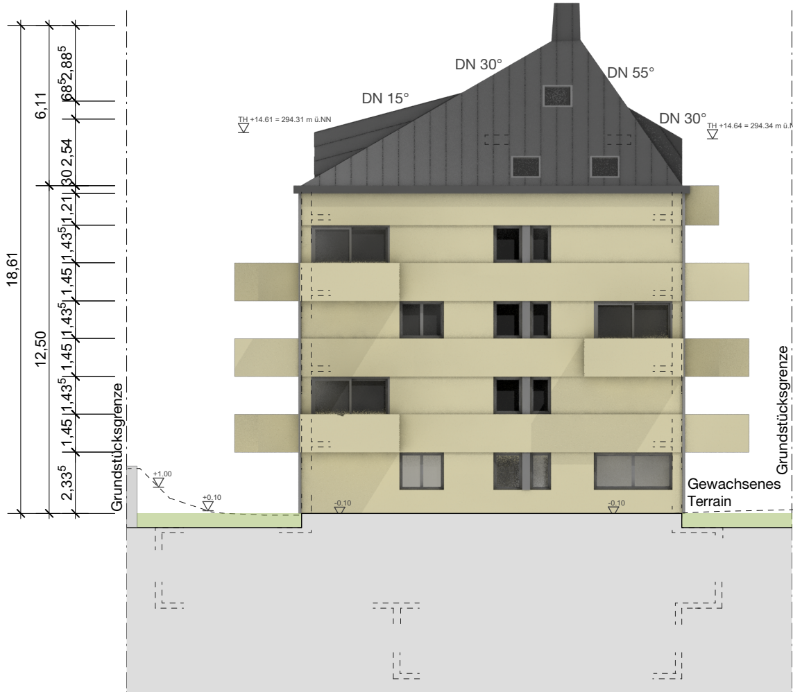
HAUS 1 ANSICHT SÜD
