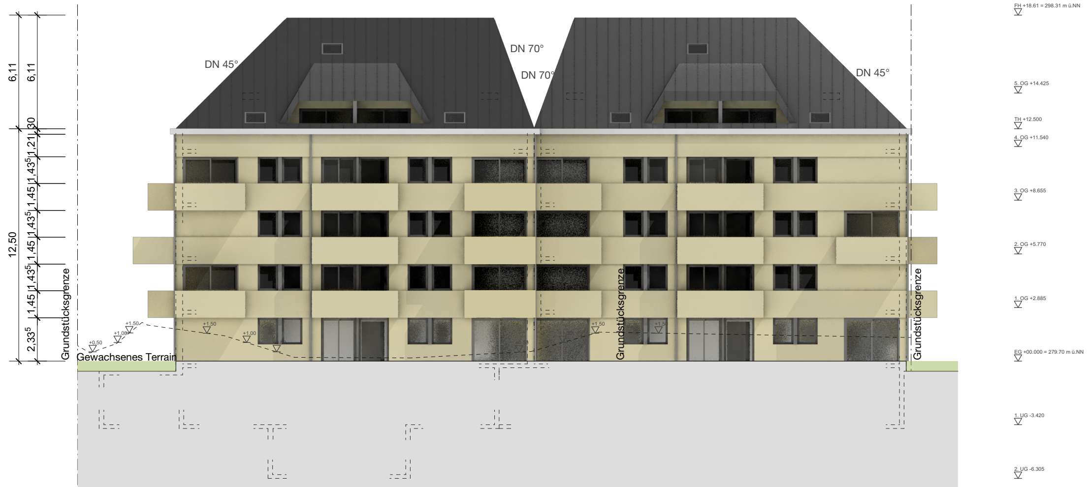
HAUS 2 - 3 ANSICHT SÜD
