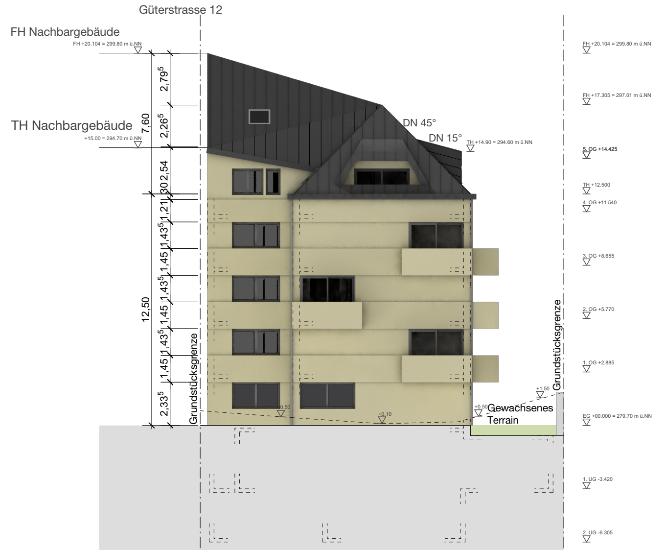
HAUS 4 ANSICHT NORD
