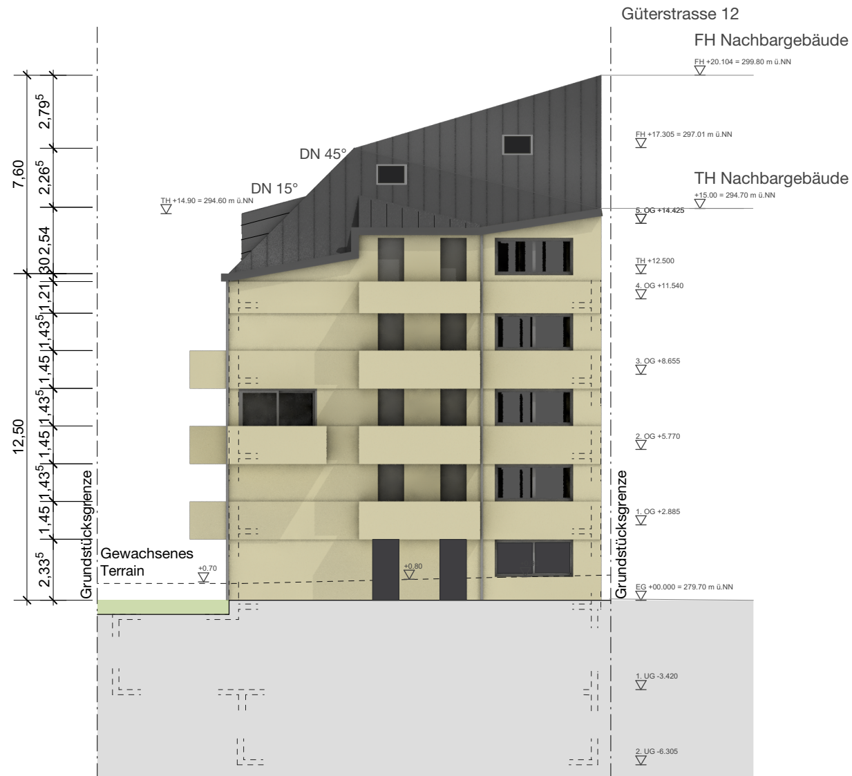
HAUS 4 ANSICHT SÜD
