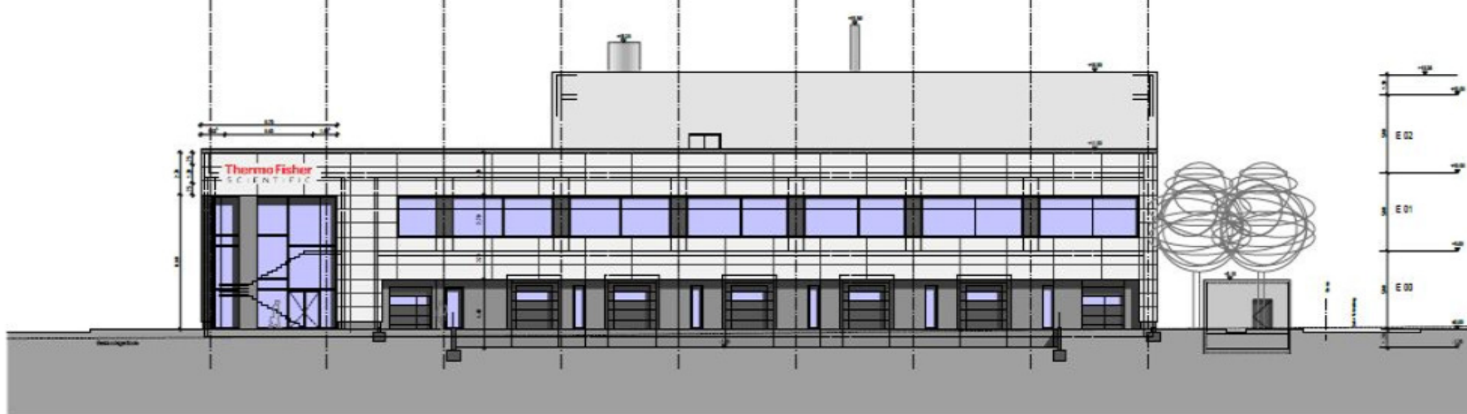
Ansicht Ost
