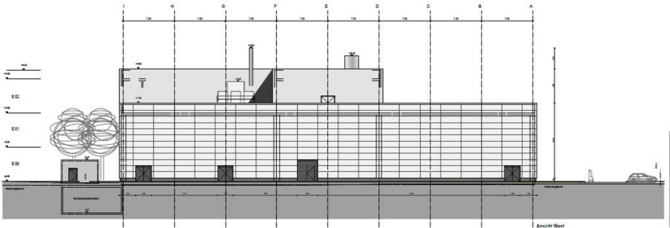
Ansicht West
