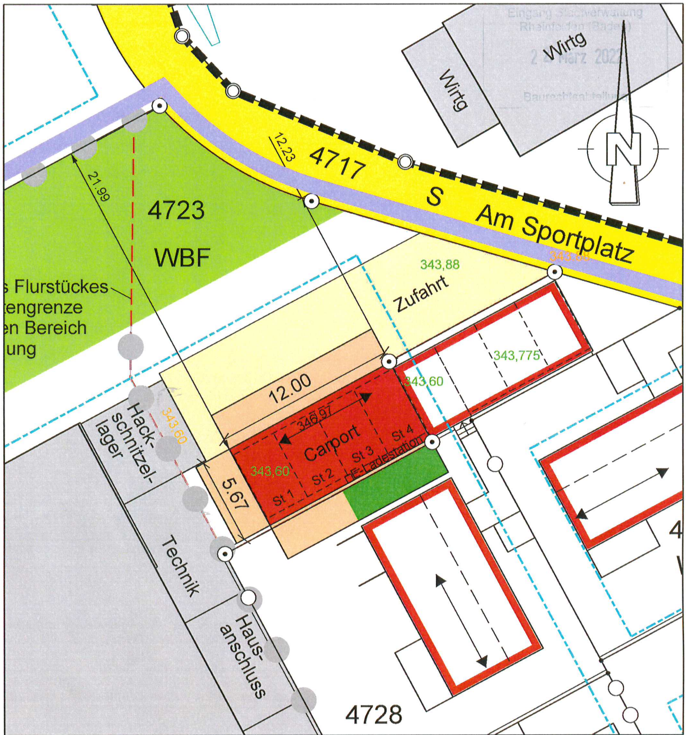
Abstandsflächenplan M 1:250 n. § 5 Abs. 7 LBO
