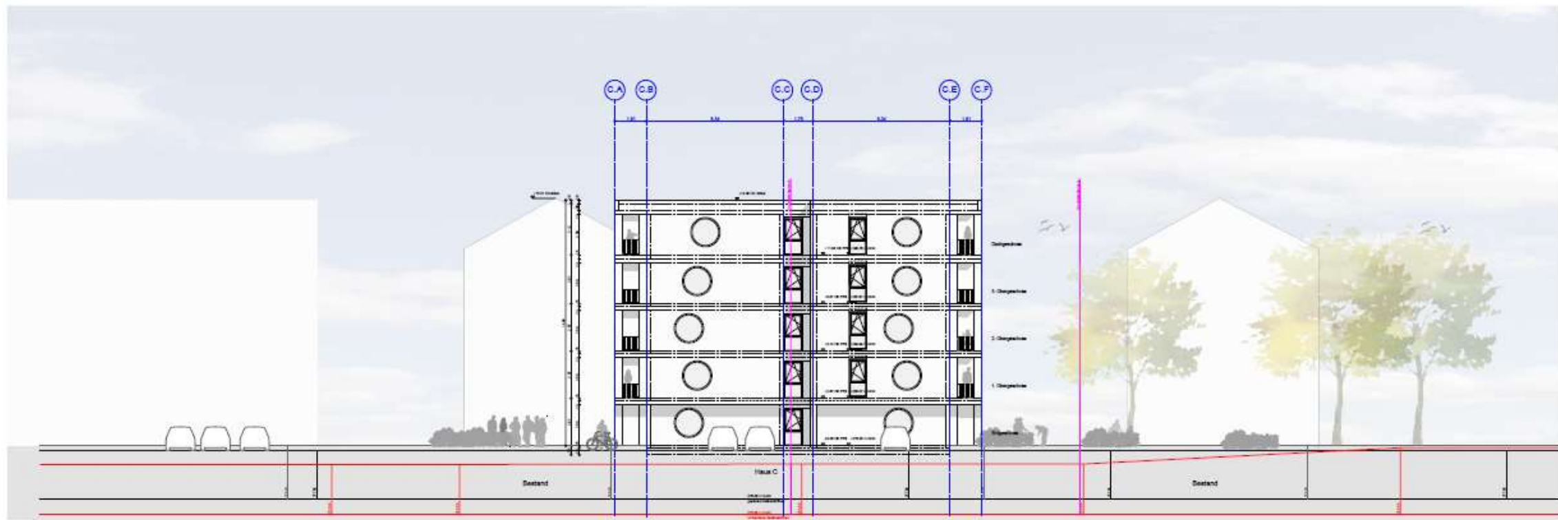
Ansicht Süd
